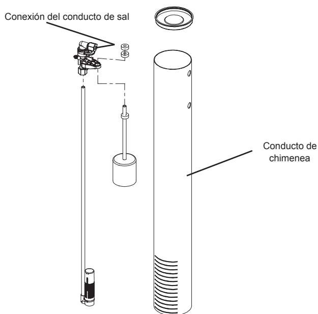
Figura 14 Conjunto aspiración de salmuera
