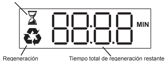
Figura 17 Pantalla durante la regeneración.
