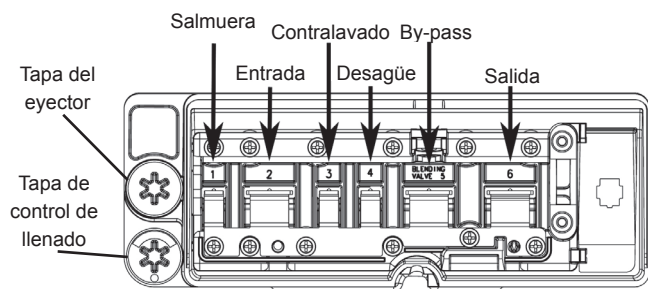
Figura 23 Diseño de la válvula
