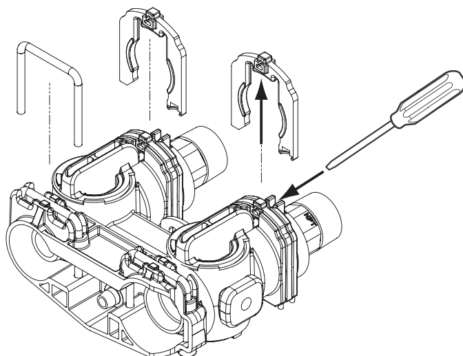
Figura 10 Conjunto del by-pass
