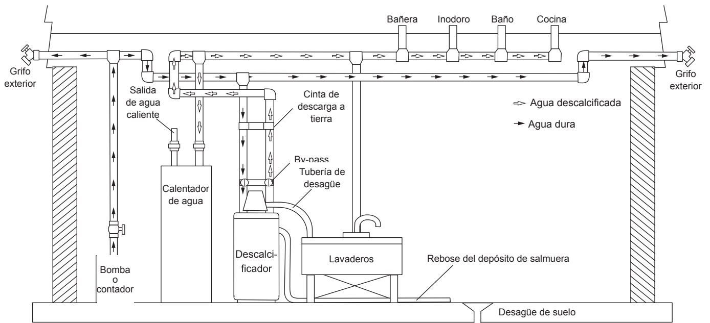
Figura 7 Diagrama de flujo de agua descalcificada
