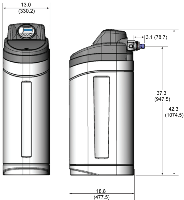
Figura 5 Dimensiones
