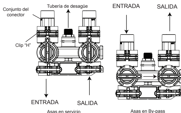
Figura 9 Serie 360 operación de by-pass
